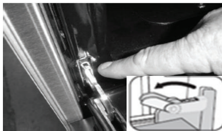
Cerniera bloccabile
